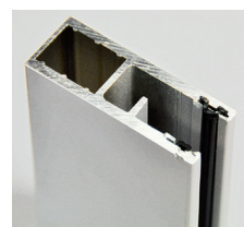
coulisse 67x25
